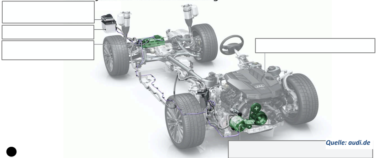
Mild-Hybrid 48 Volt-Antriebsstrang
