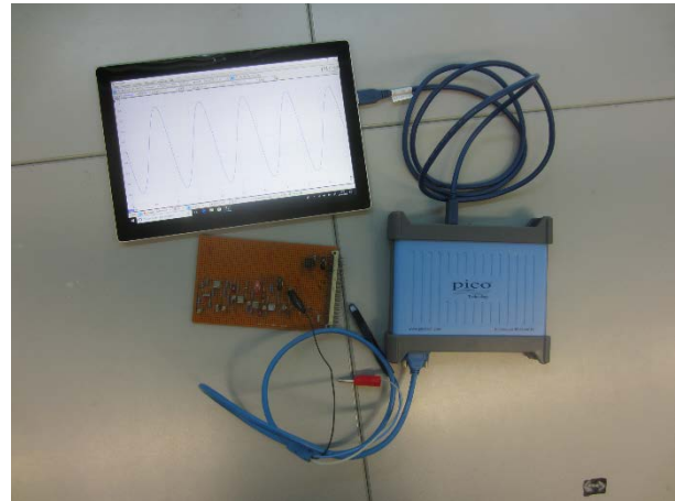
PC-Oszilloskop
